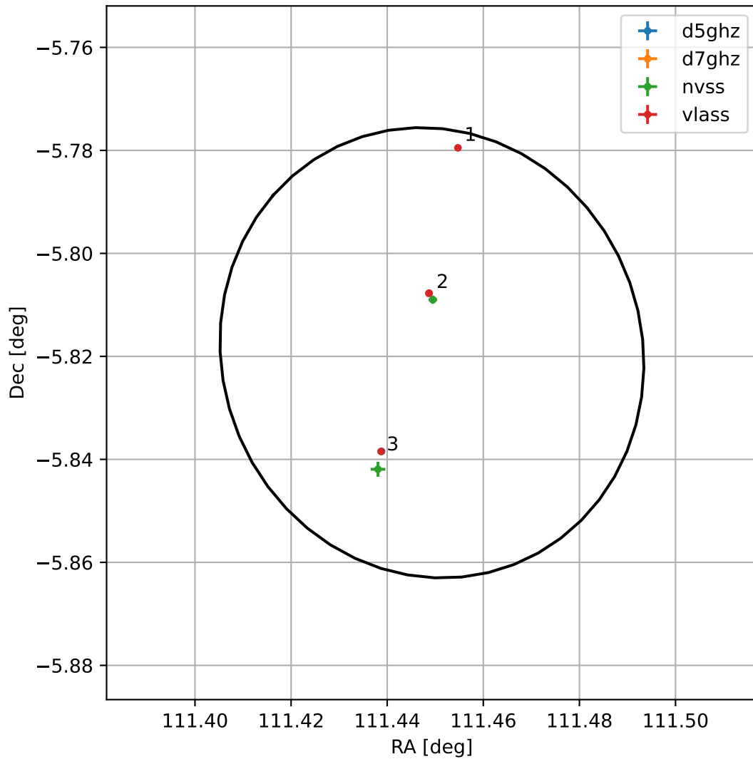
4FGL J0725.7-0549
