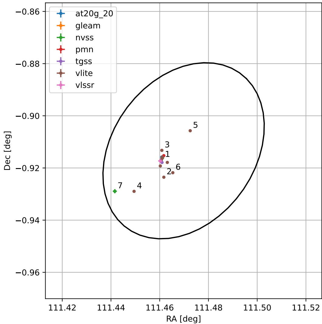
4FGL J0725.8-0054
