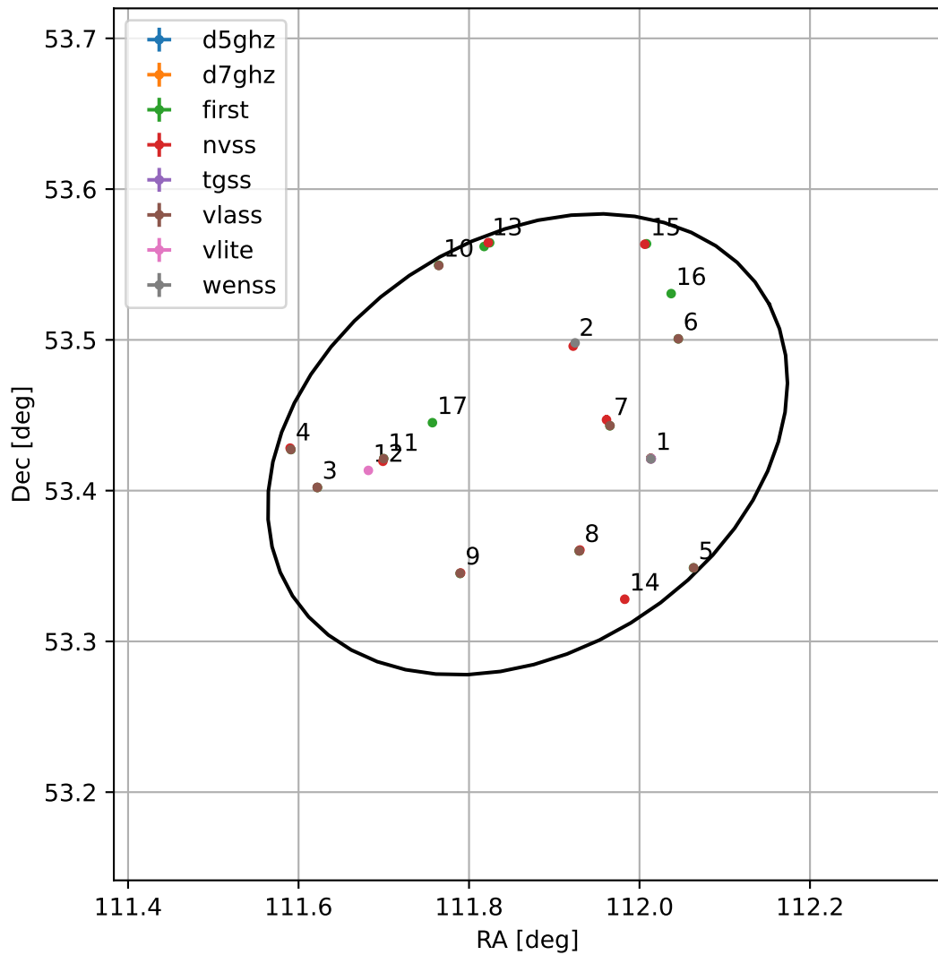
4FGL J0727.4+5325
