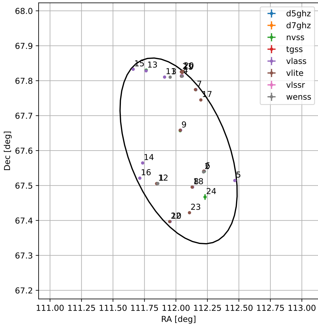
4FGL J0728.0+6735
