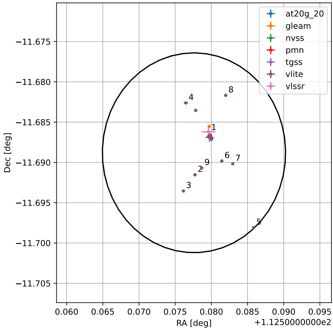
4FGL J0730.3-1141
