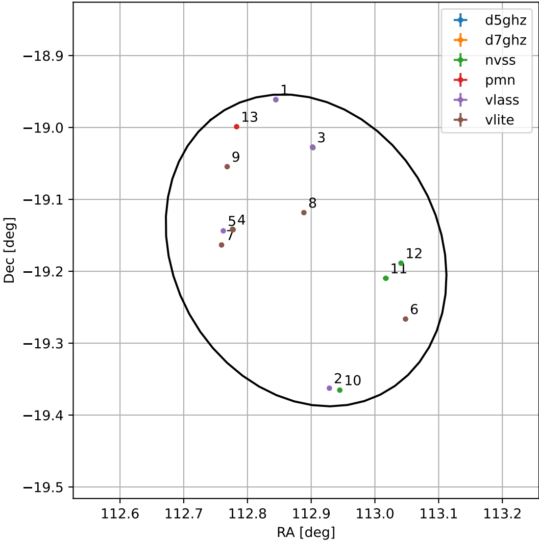
4FGL J0731.5-1910
