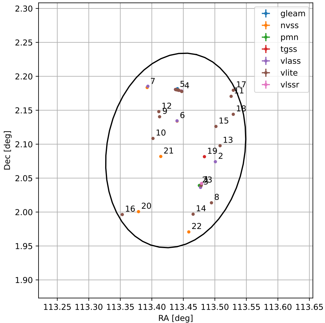
4FGL J0733.7+0205
