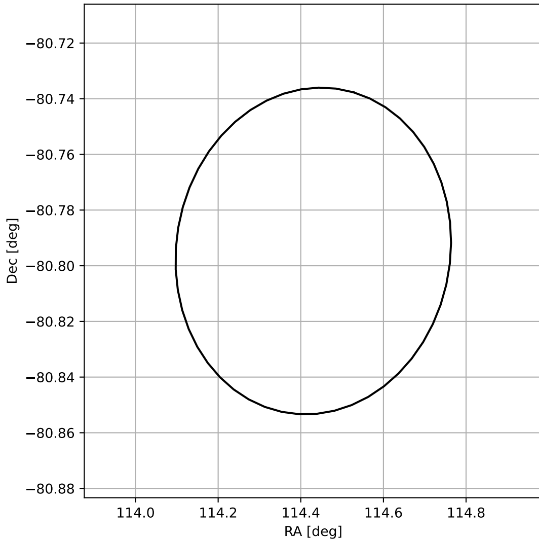
4FGL J0737.7-8047
