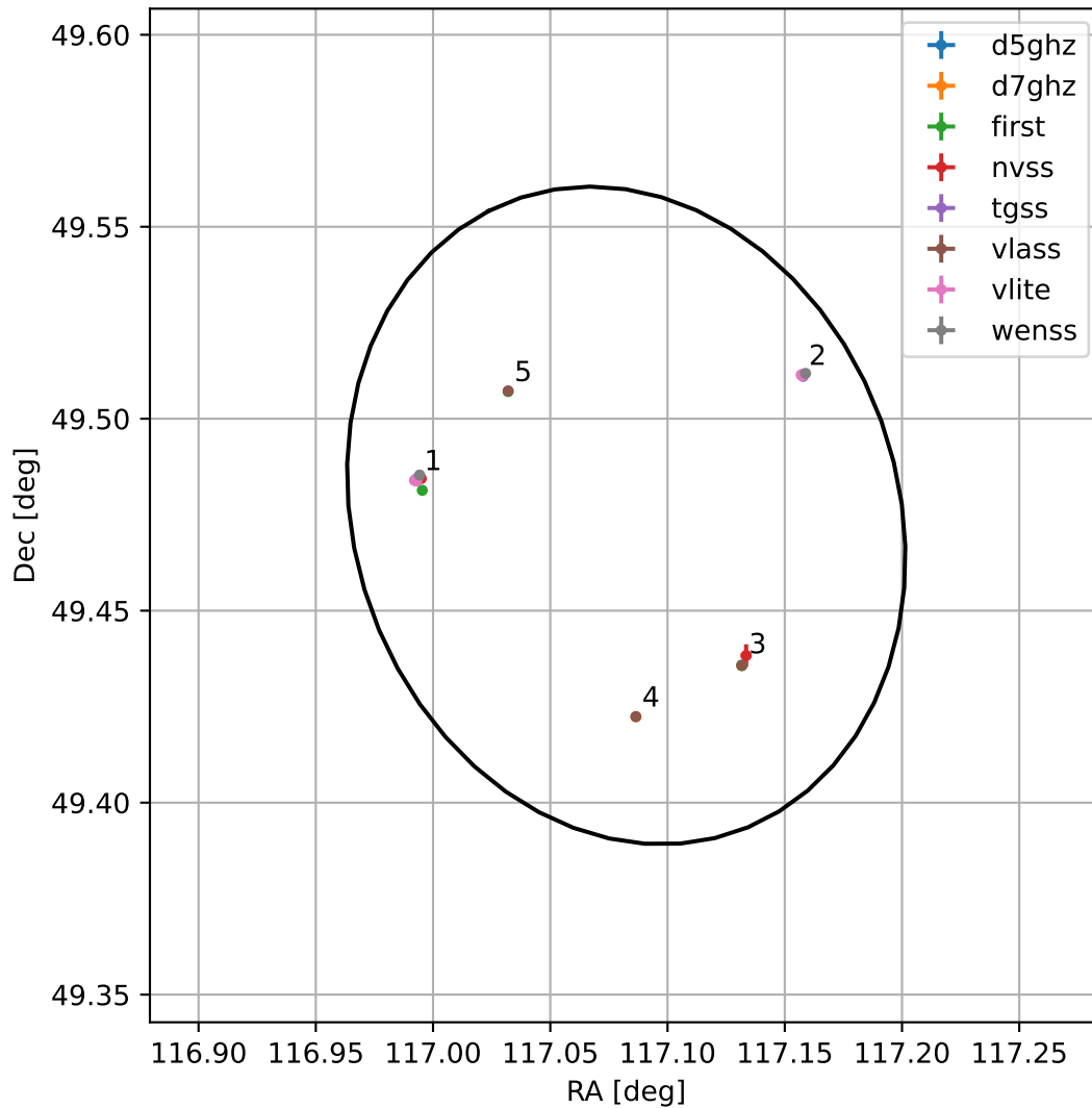
4FGL J0748.3+4928
