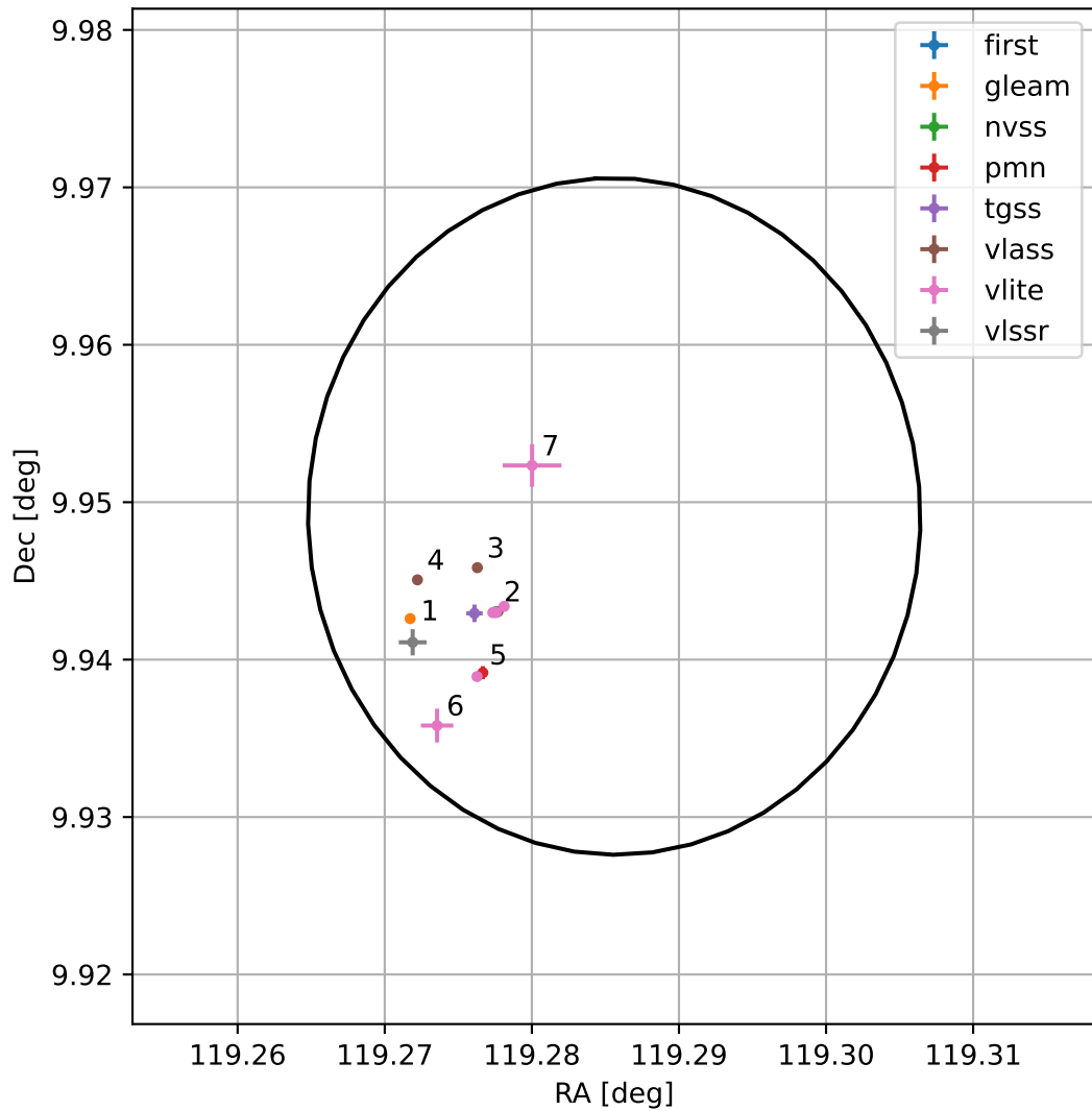
4FGL J0757.1+0956
