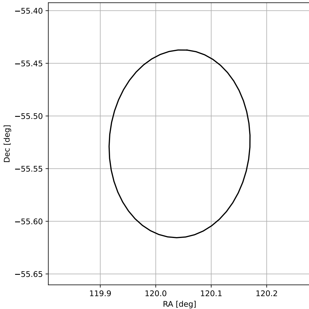
4FGL J0800.1-5531
