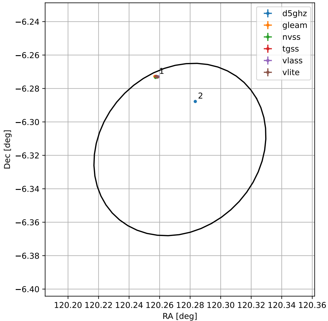
4FGL J0801.0-0618
