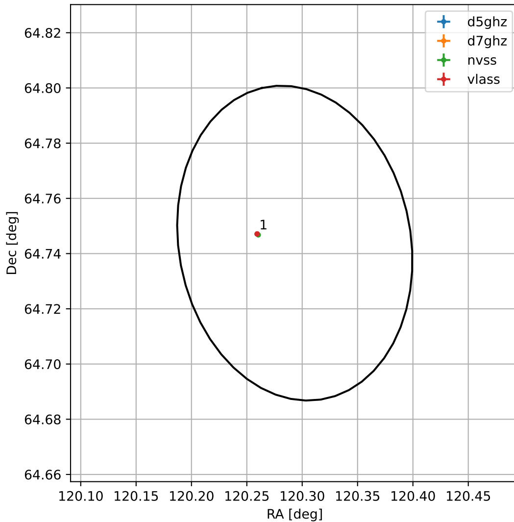
4FGL J0801.1+6444
