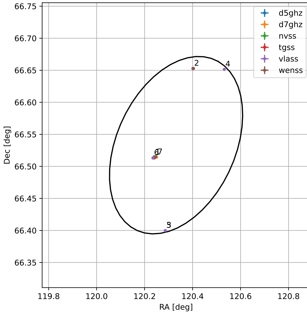
4FGL J0801.3+6631
