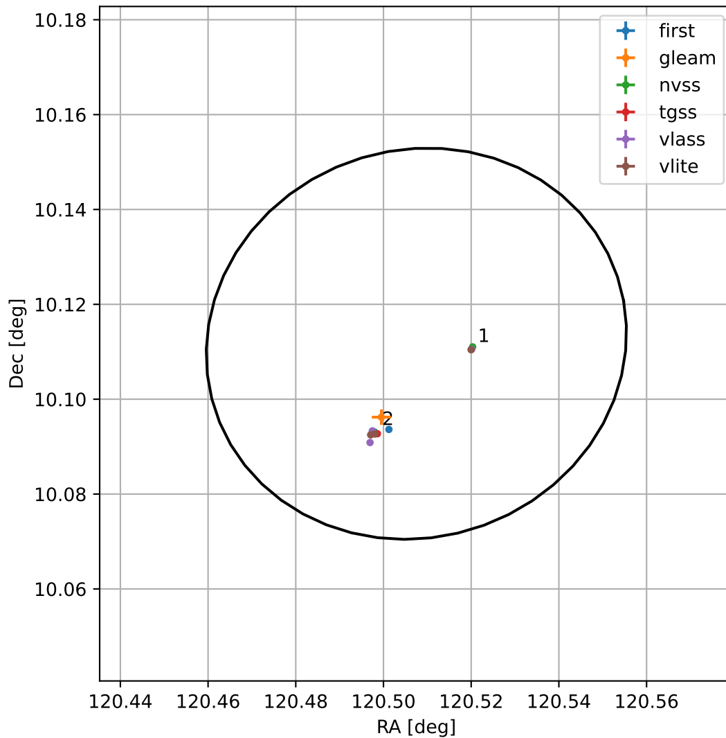
4FGL J0802.0+1006
