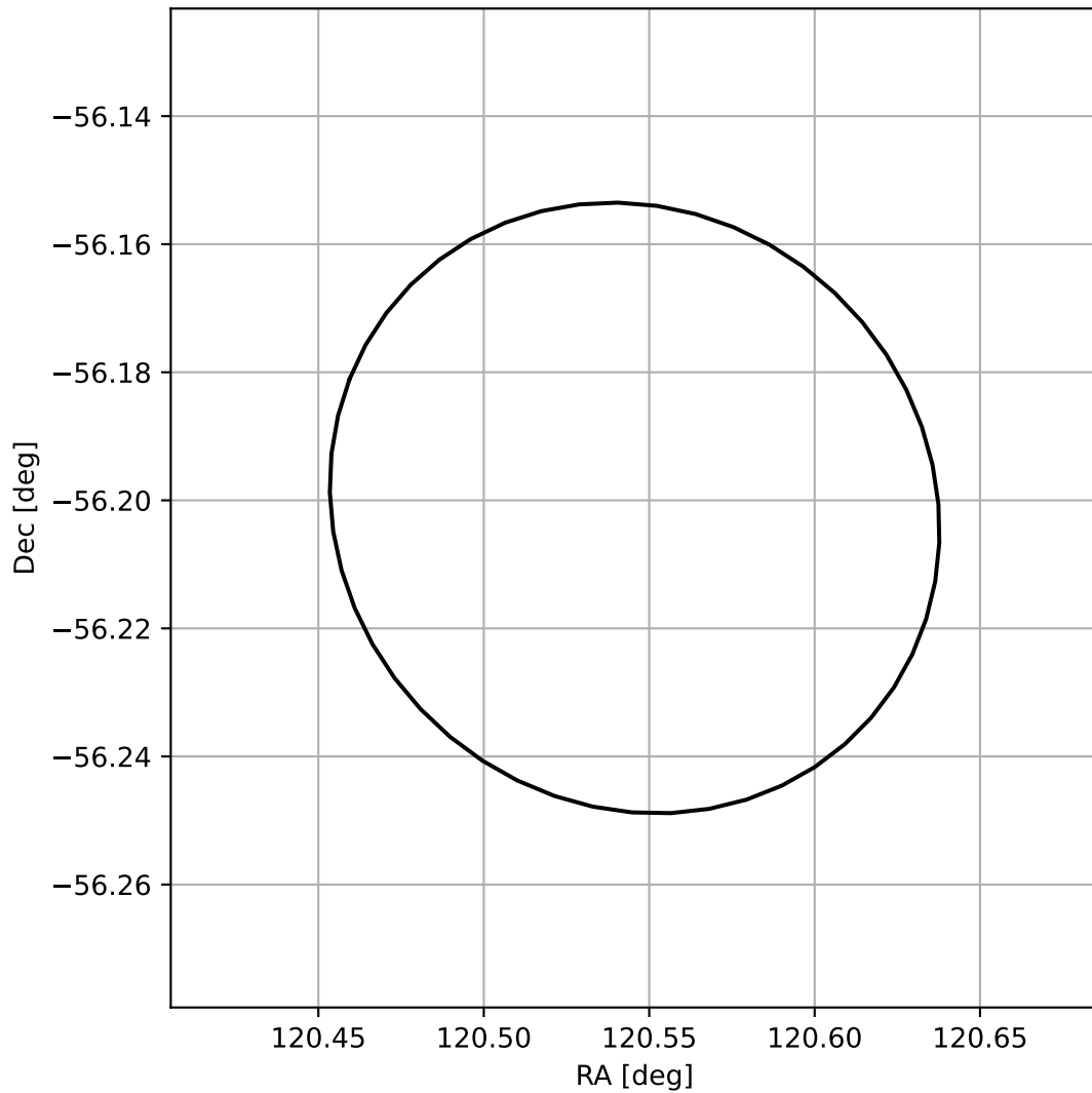
4FGL J0802.1-5612
