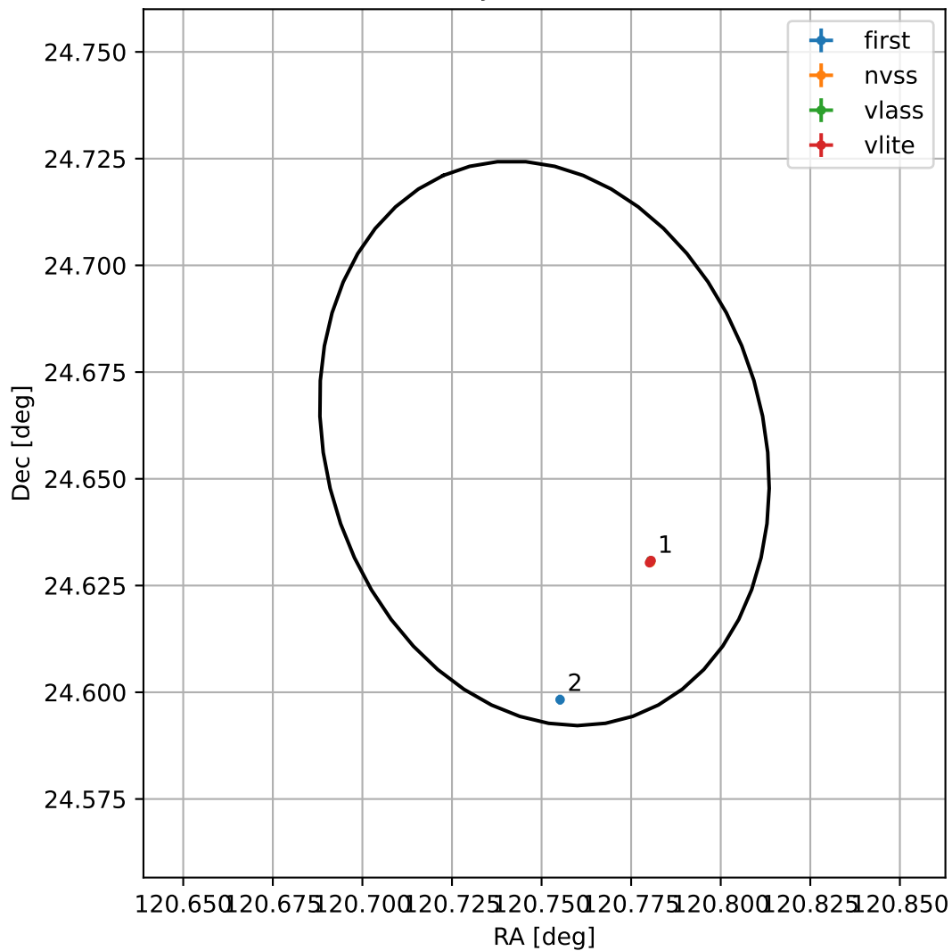
4FGL J0803.0+2439
