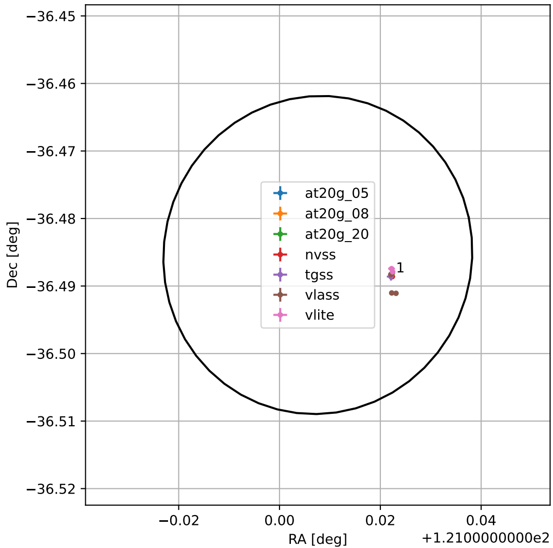
4FGL J0804.0-3629
