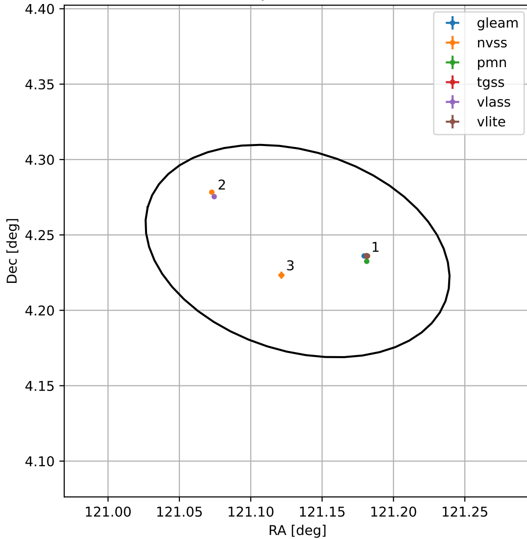
4FGL J0804.5+0414
