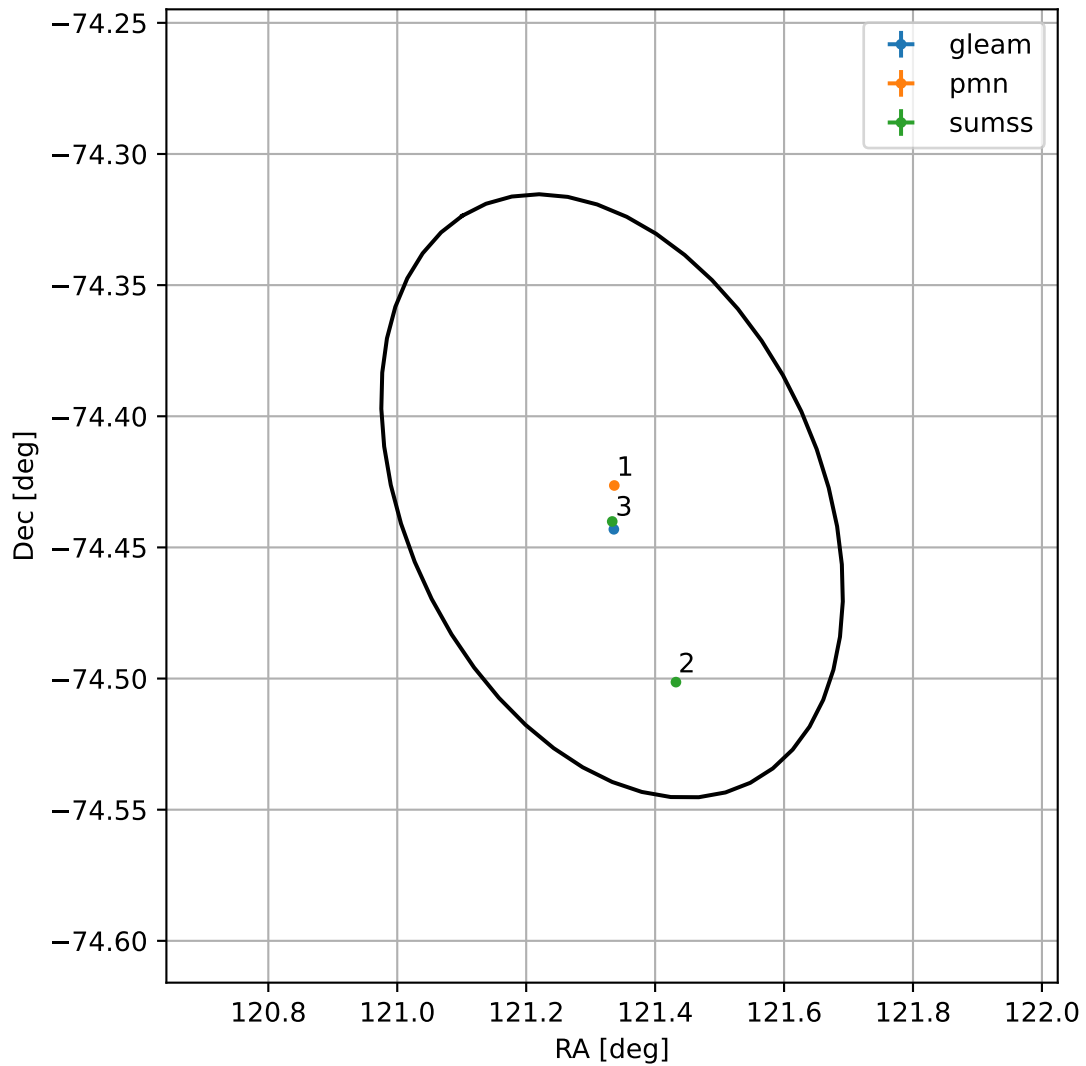
4FGL J0805.3-7425
