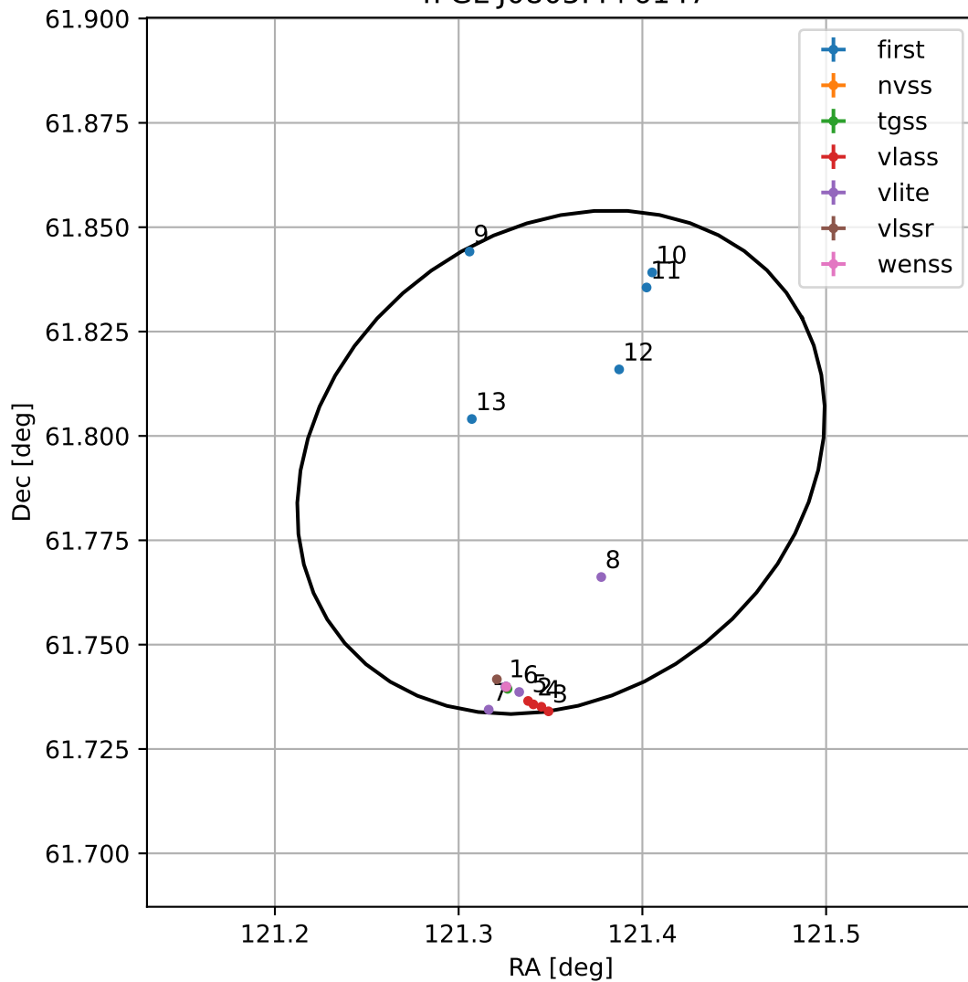
4FGL J0805.4+6147
