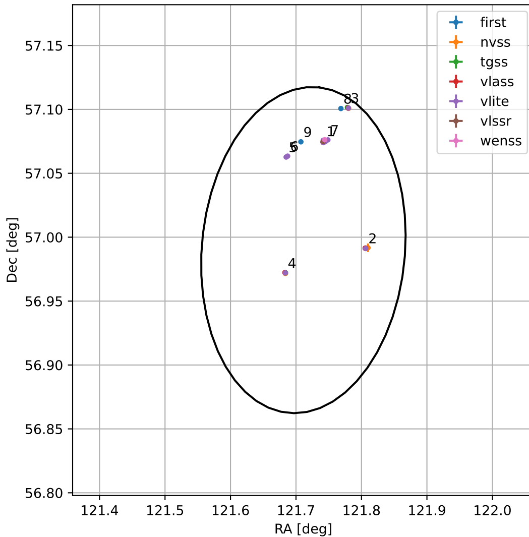
4FGL J0806.8+5659
