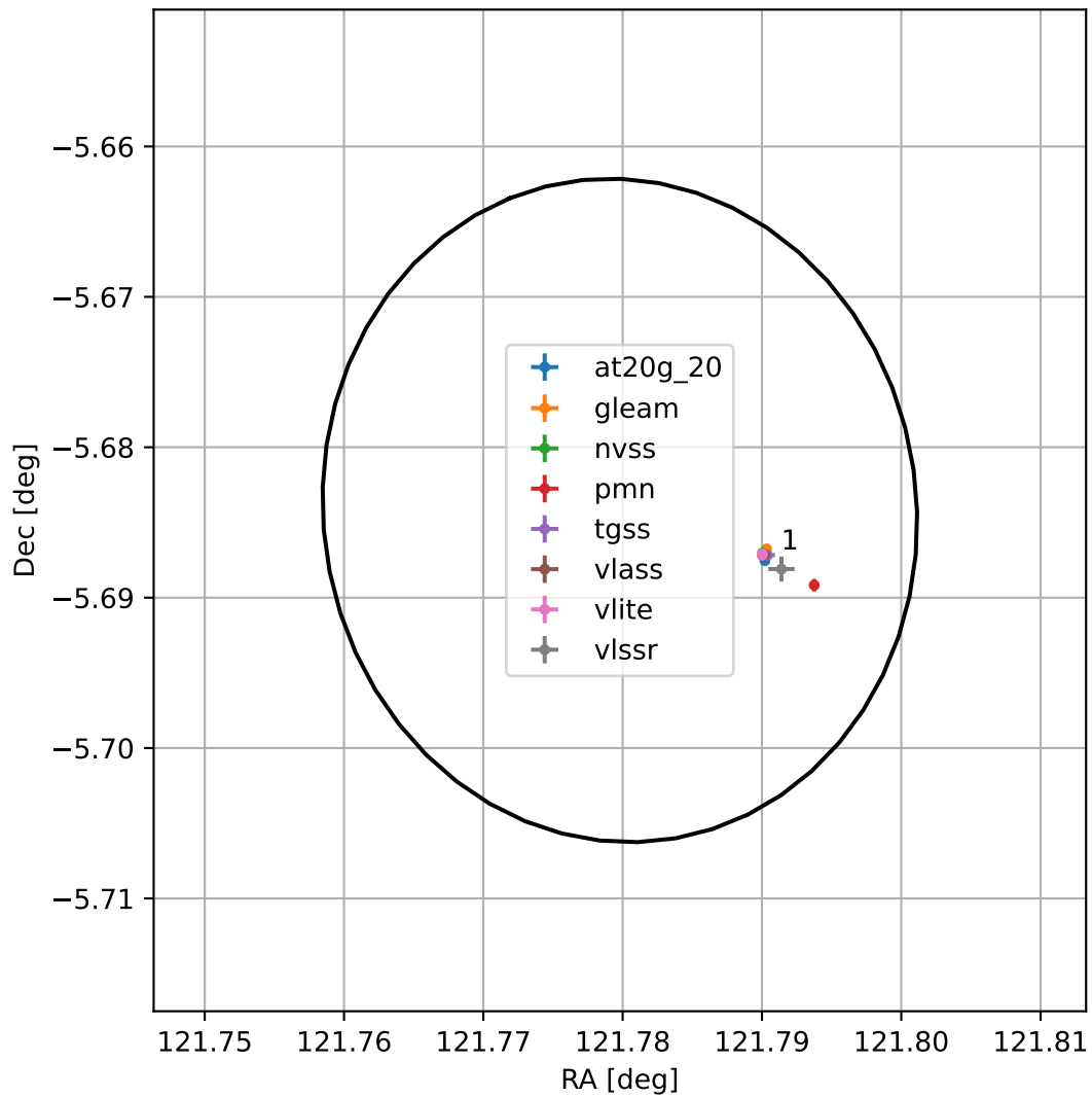
4FGL J0807.1-0541
