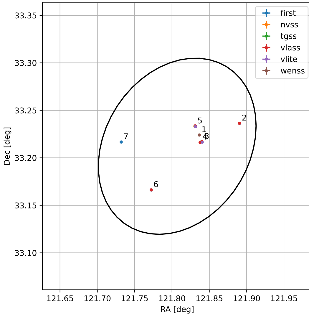
4FGL J0807.2+3312
