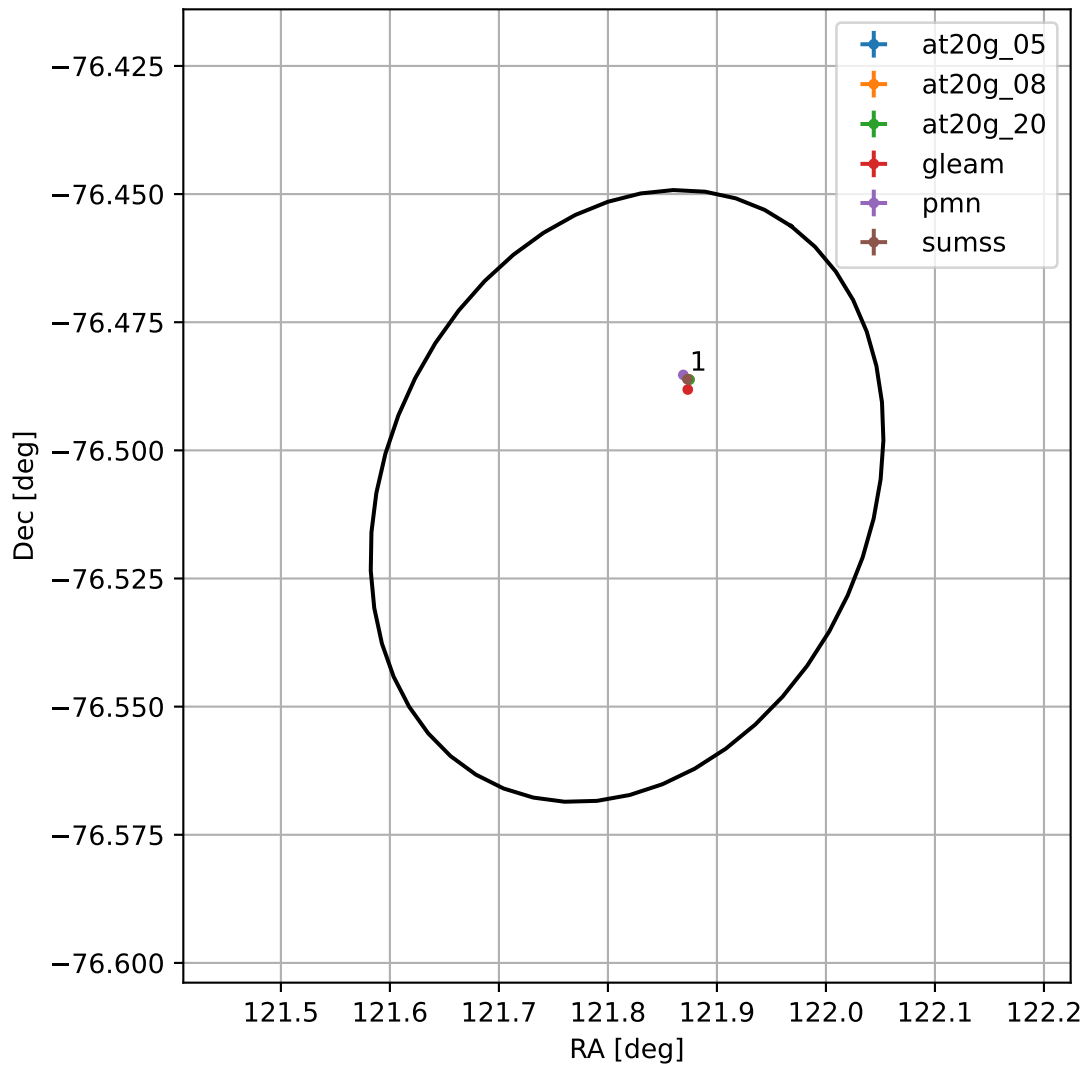
4FGL J0807.2-7630
