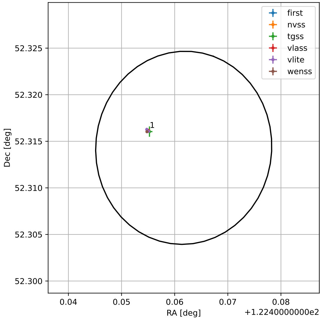
4FGL J0809.8+5218
