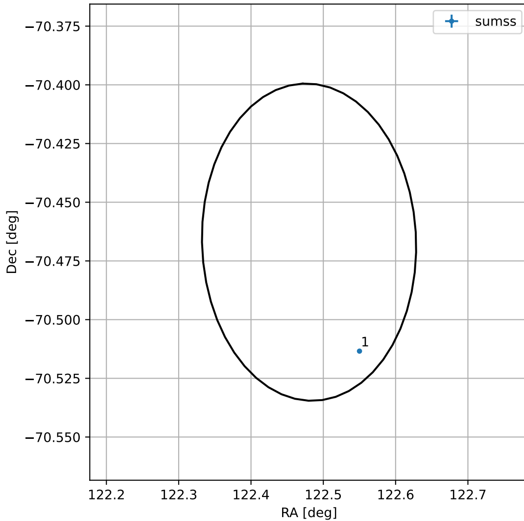
4FGL J0809.9-7028
