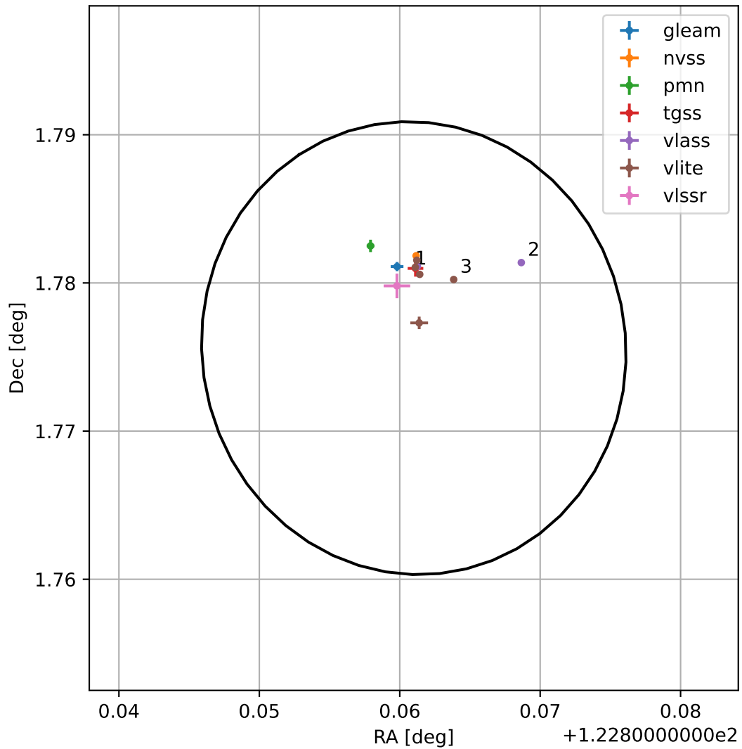
4FGL J0811.4+0146
