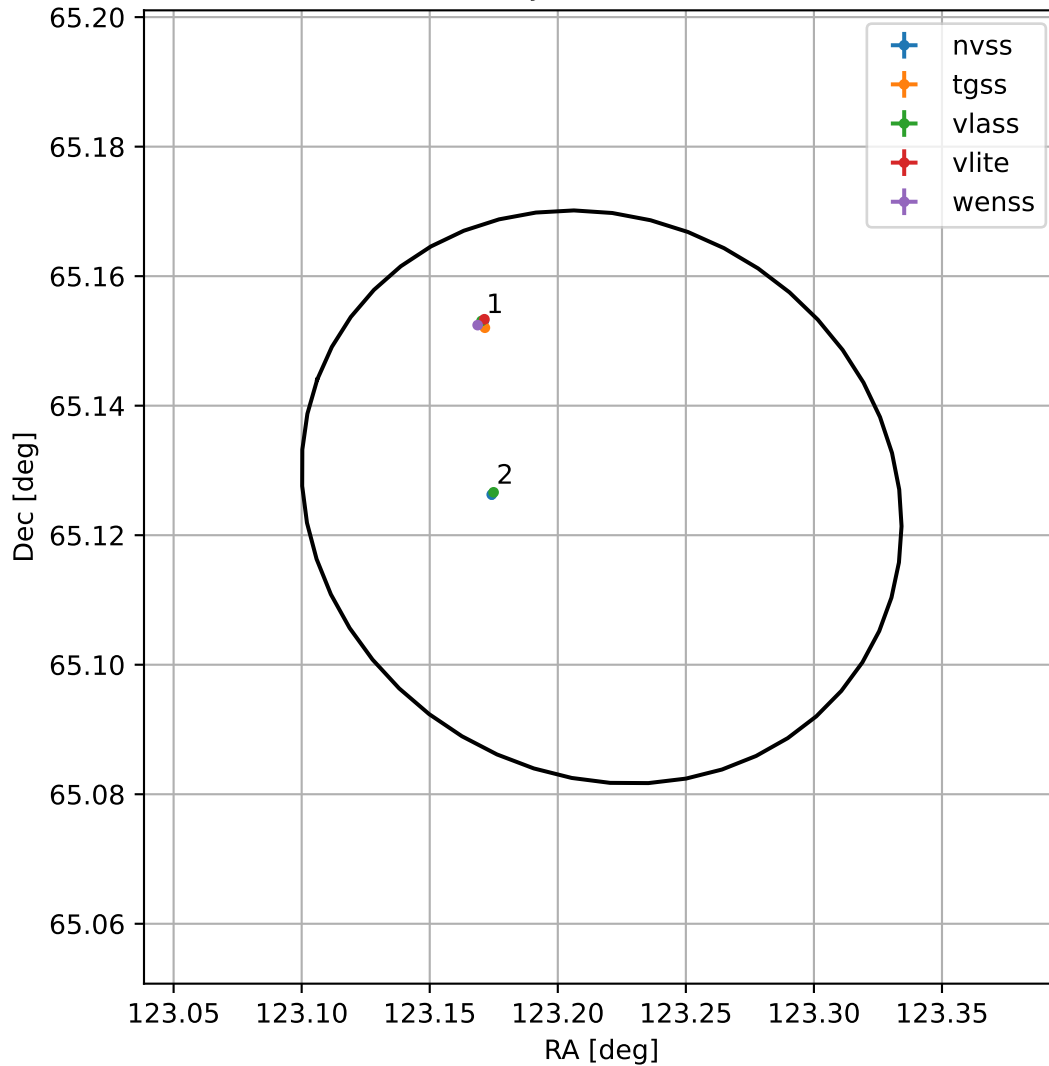
4FGL J0812.8+6507
