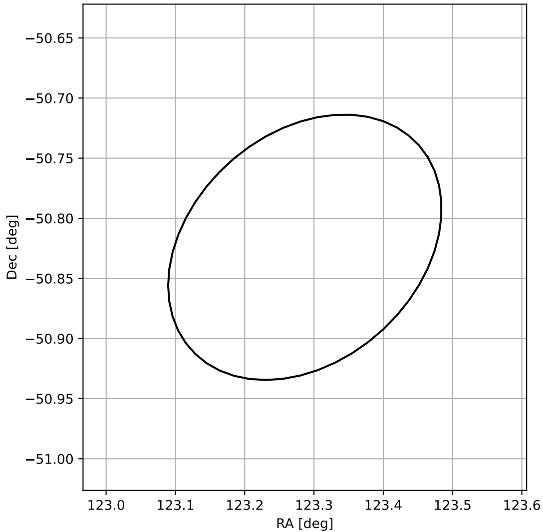
4FGL J0813.1-5049
