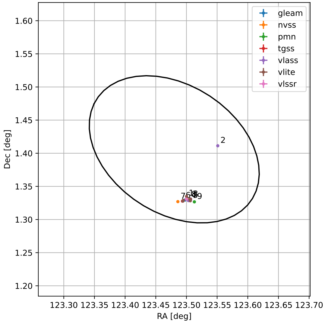
4FGL J0813.9+0124
