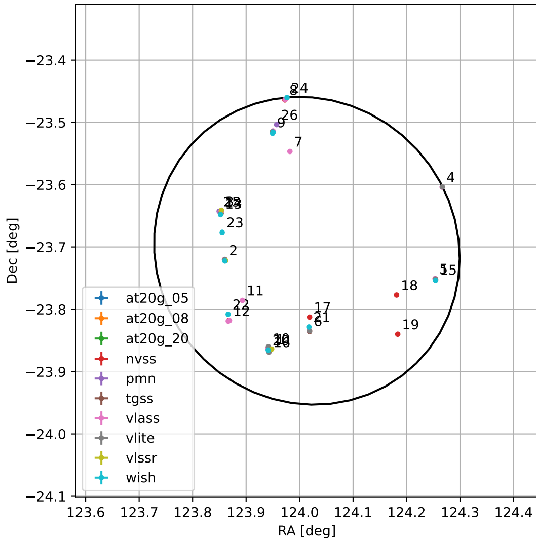
4FGL J0816.0-2342
