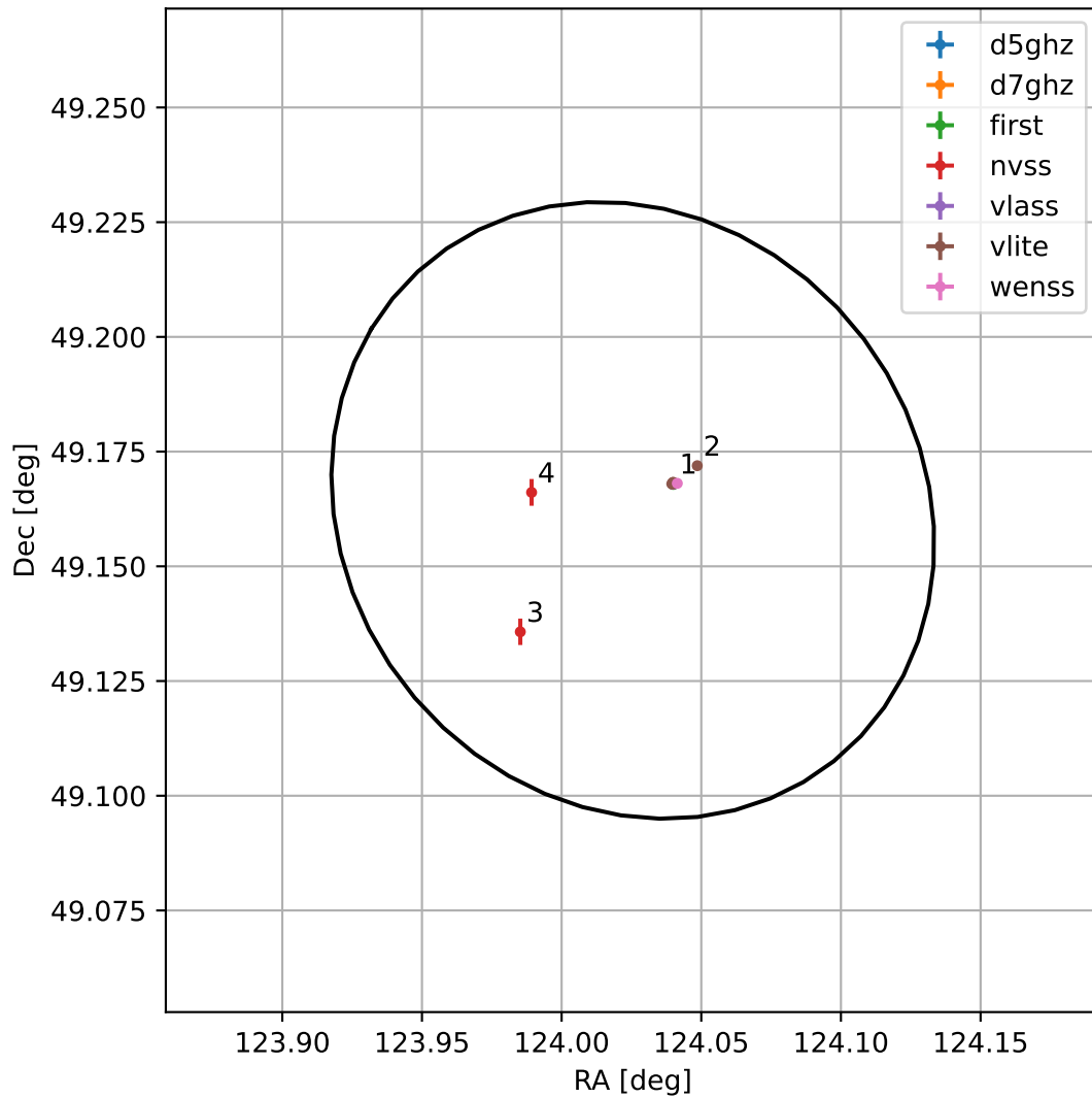
4FGL J0816.1+4909
