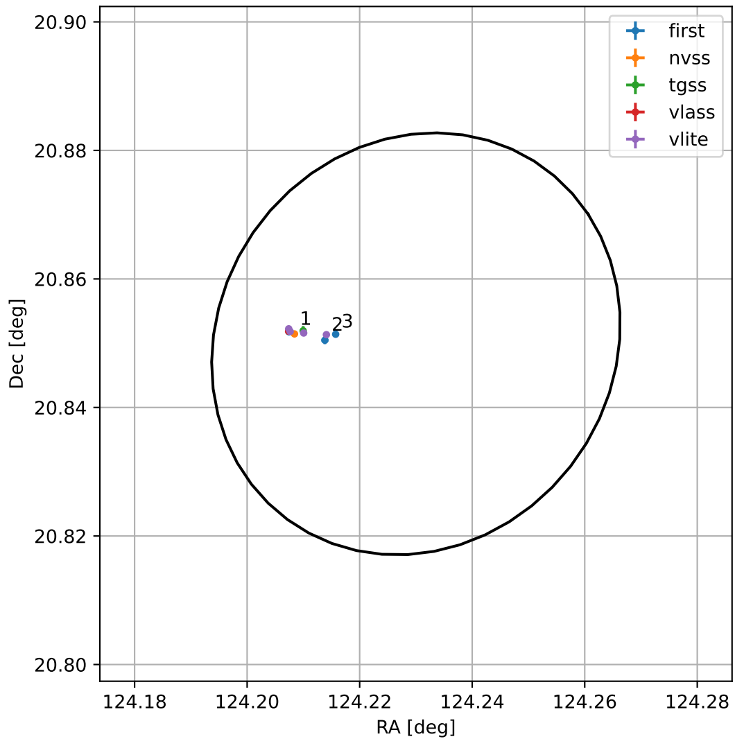
4FGL J0816.9+2050
