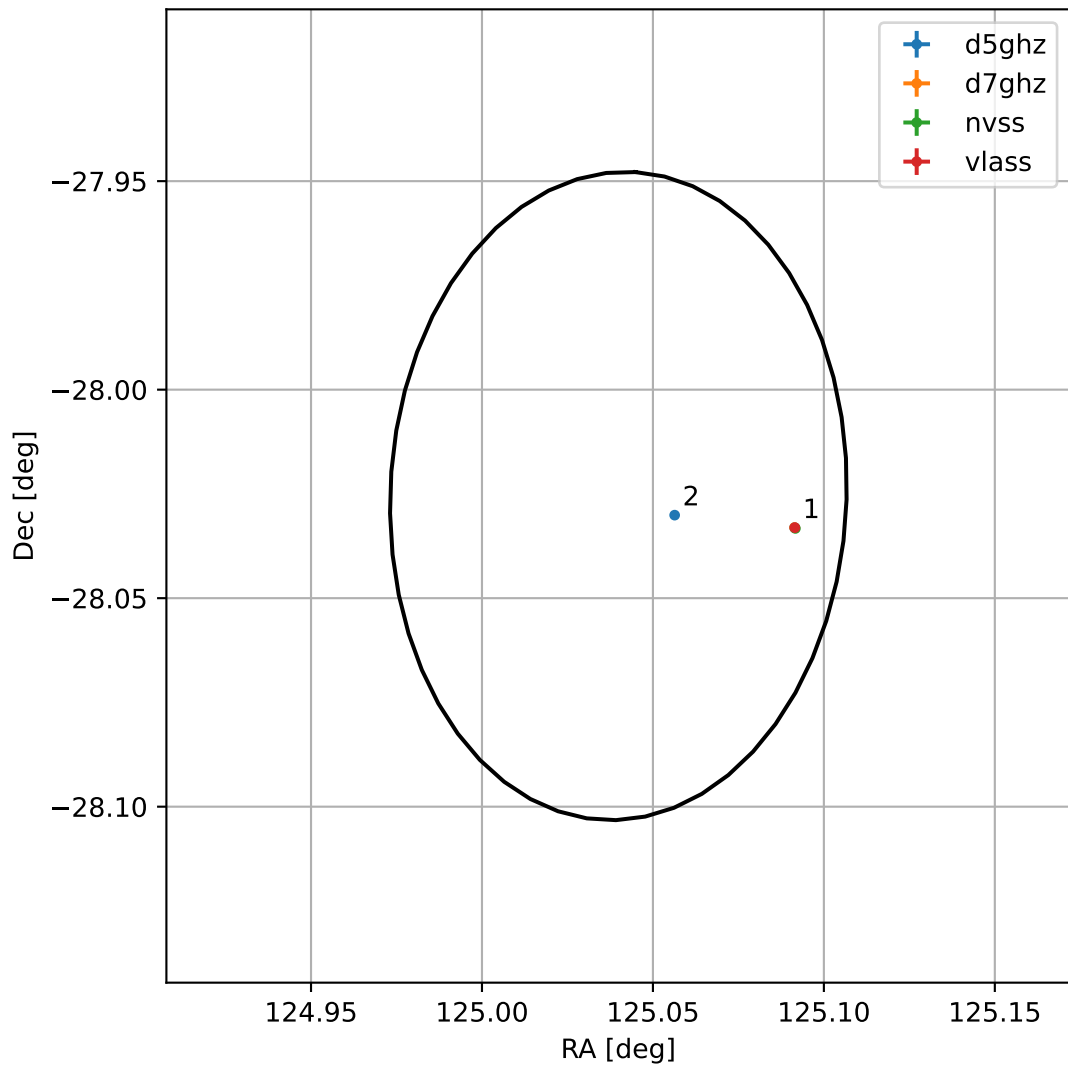
4FGL J0820.1-2801
