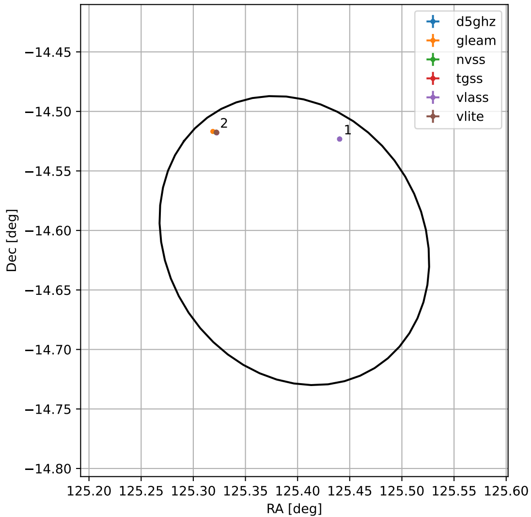
4FGL J0821.5-1436
