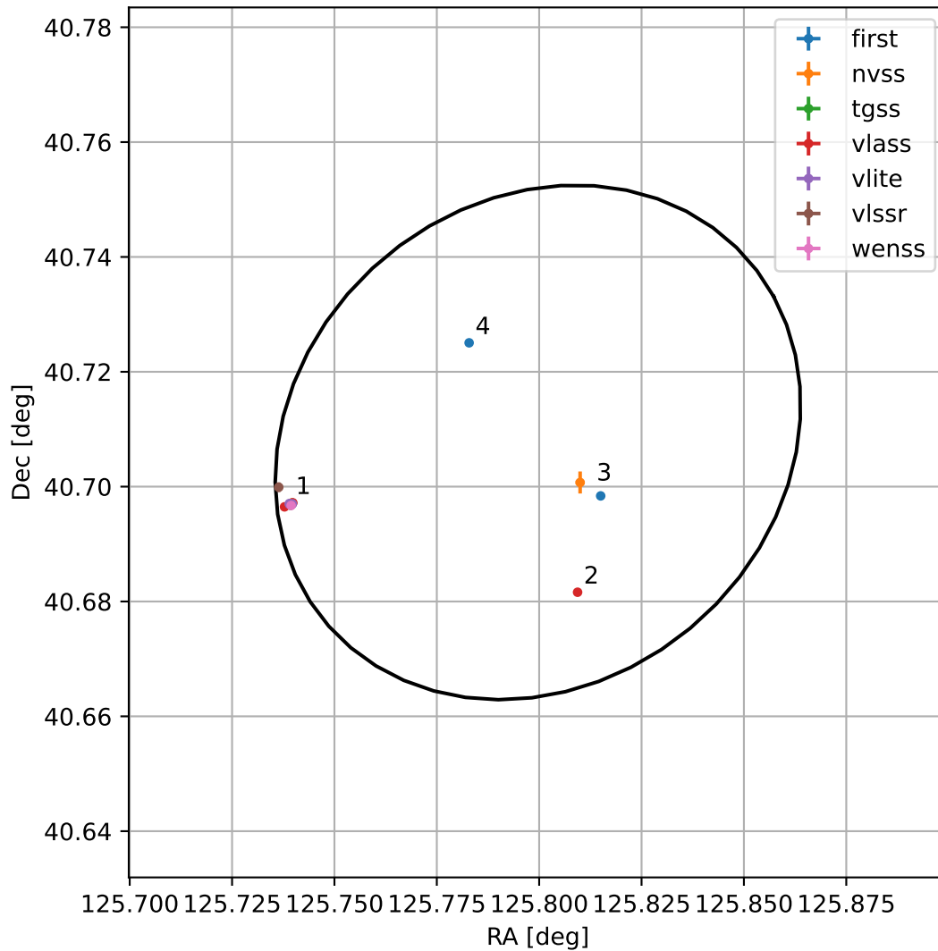
4FGL J0823.1+4042
