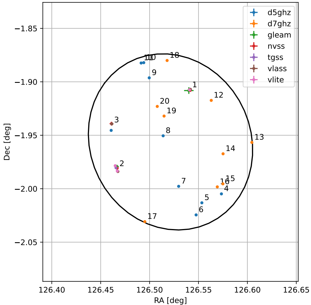
4FGL J0826.0-0157
