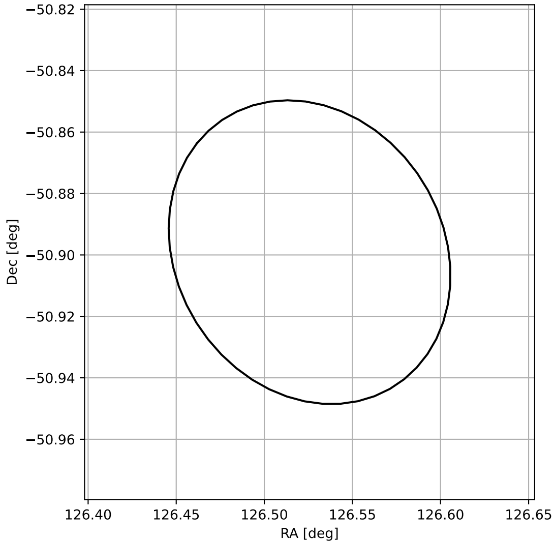
4FGL J0826.1-5053
