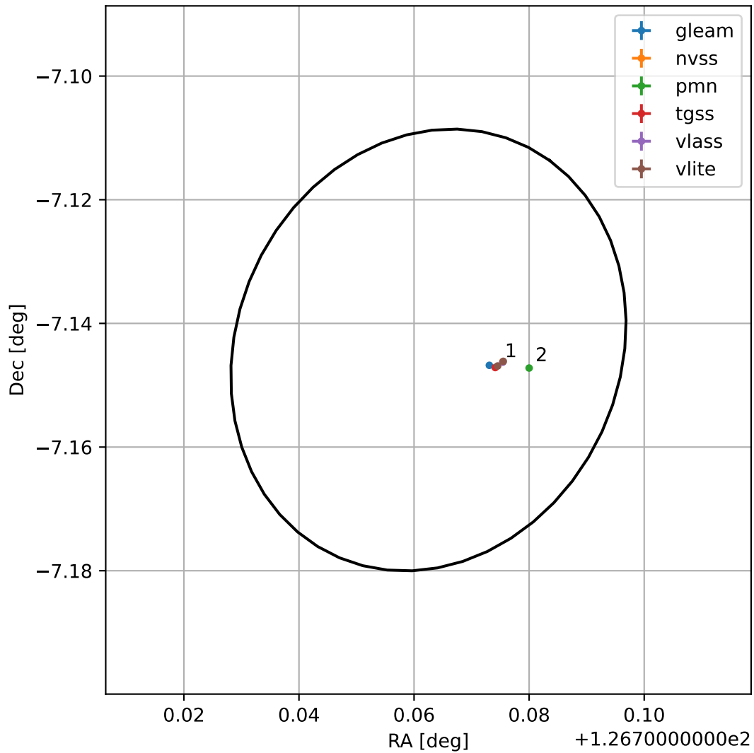
4FGL J0827.0-0708
