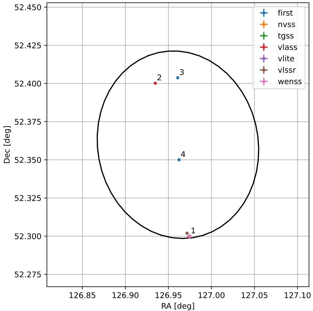
4FGL J0827.8+5221
