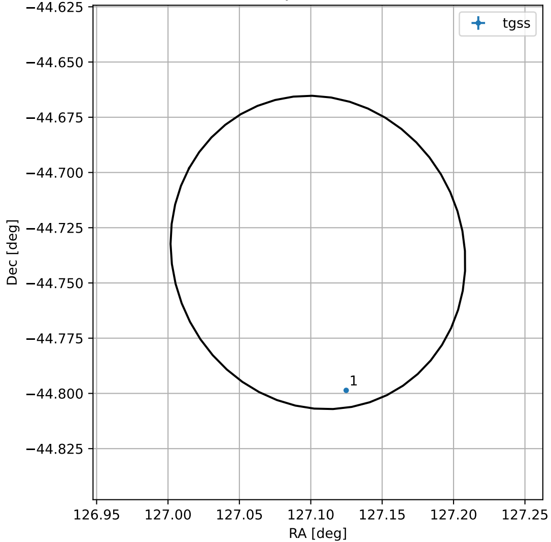
4FGL J0828.4-4444
