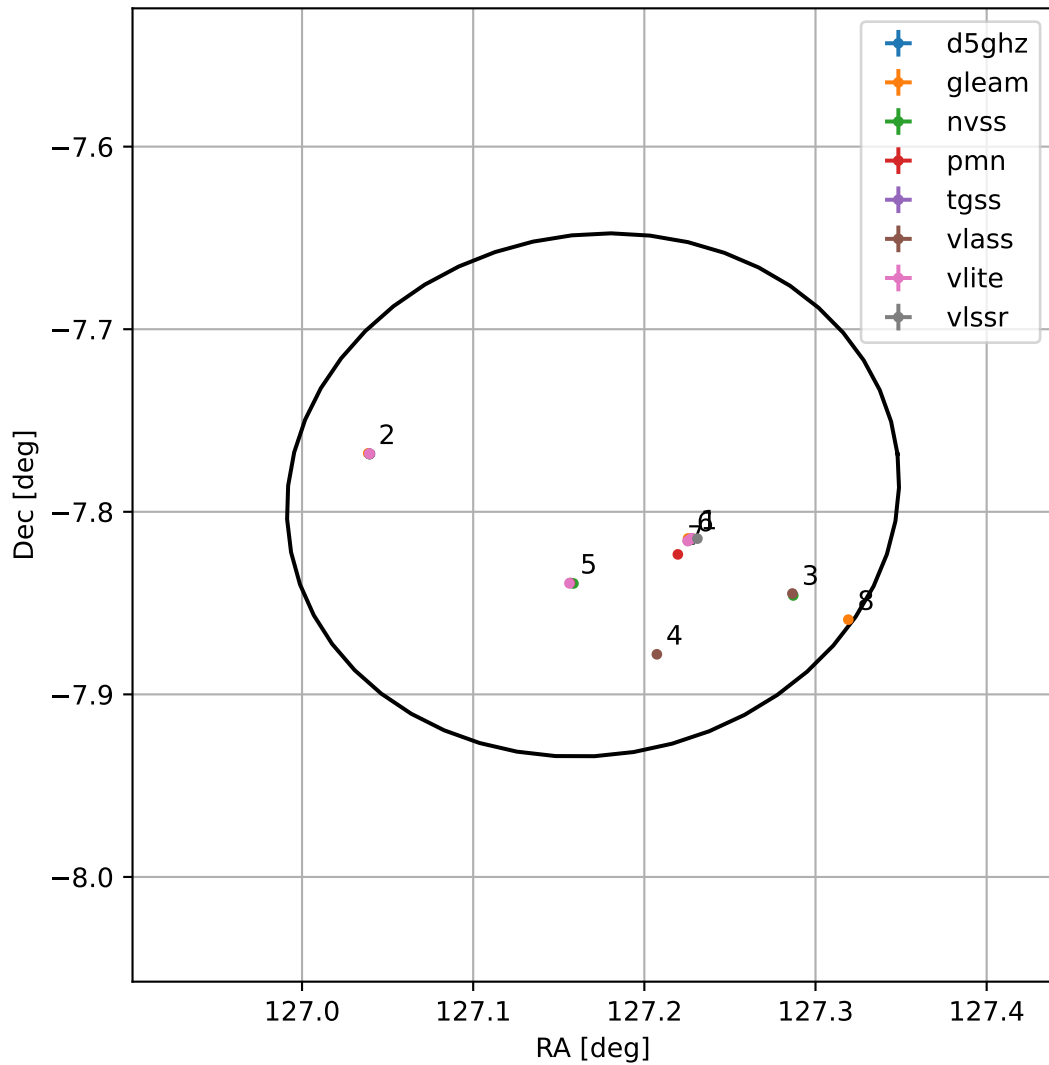
4FGL J0828.6-0747
