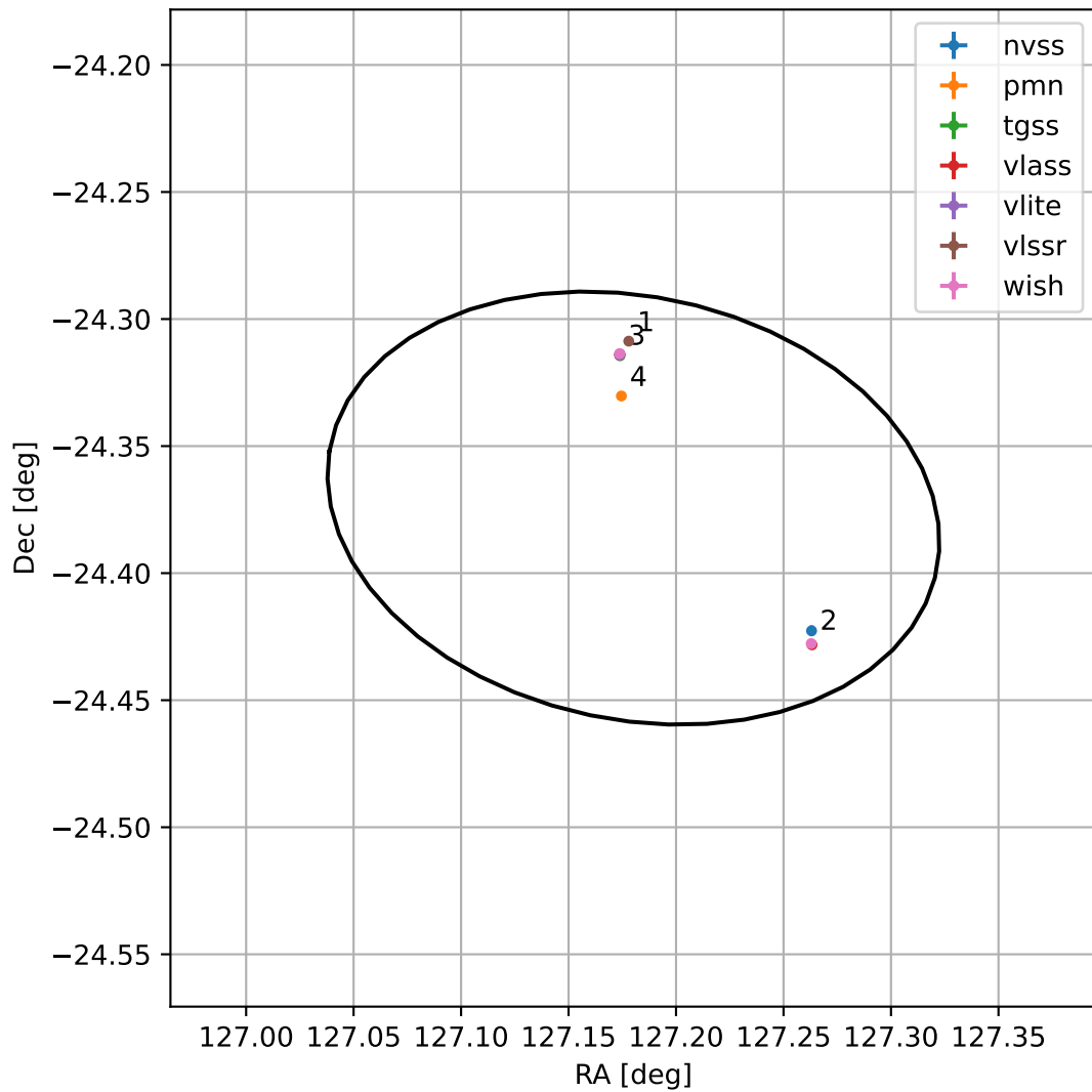
4FGL J0828.7-2422
