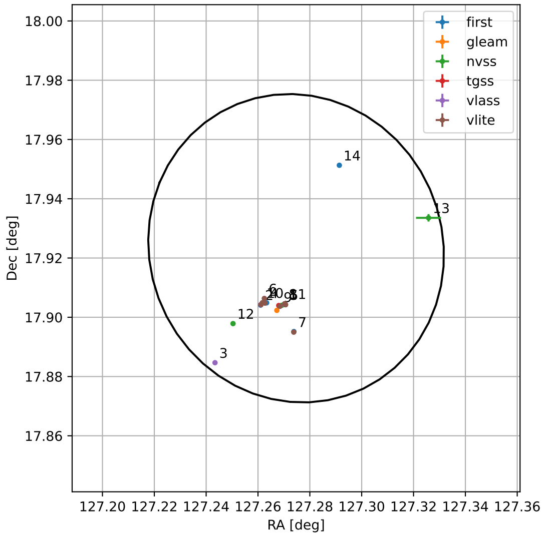
4FGL J0829.0+1755
