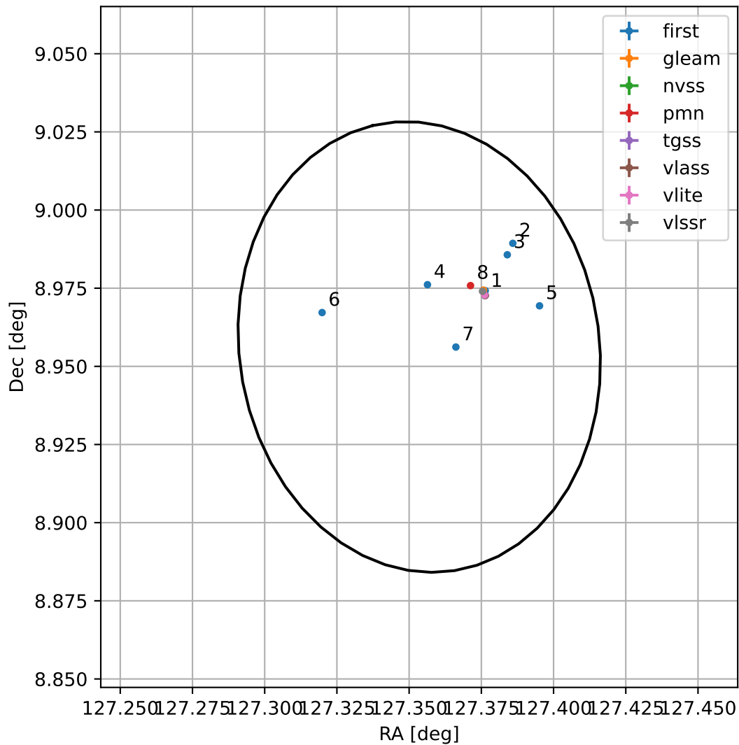
4FGL J0829.4+0857
