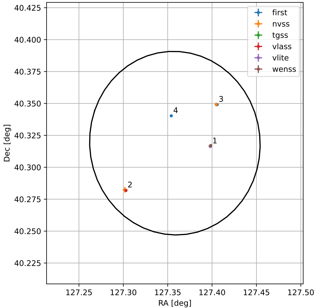
4FGL J0829.4+4019
