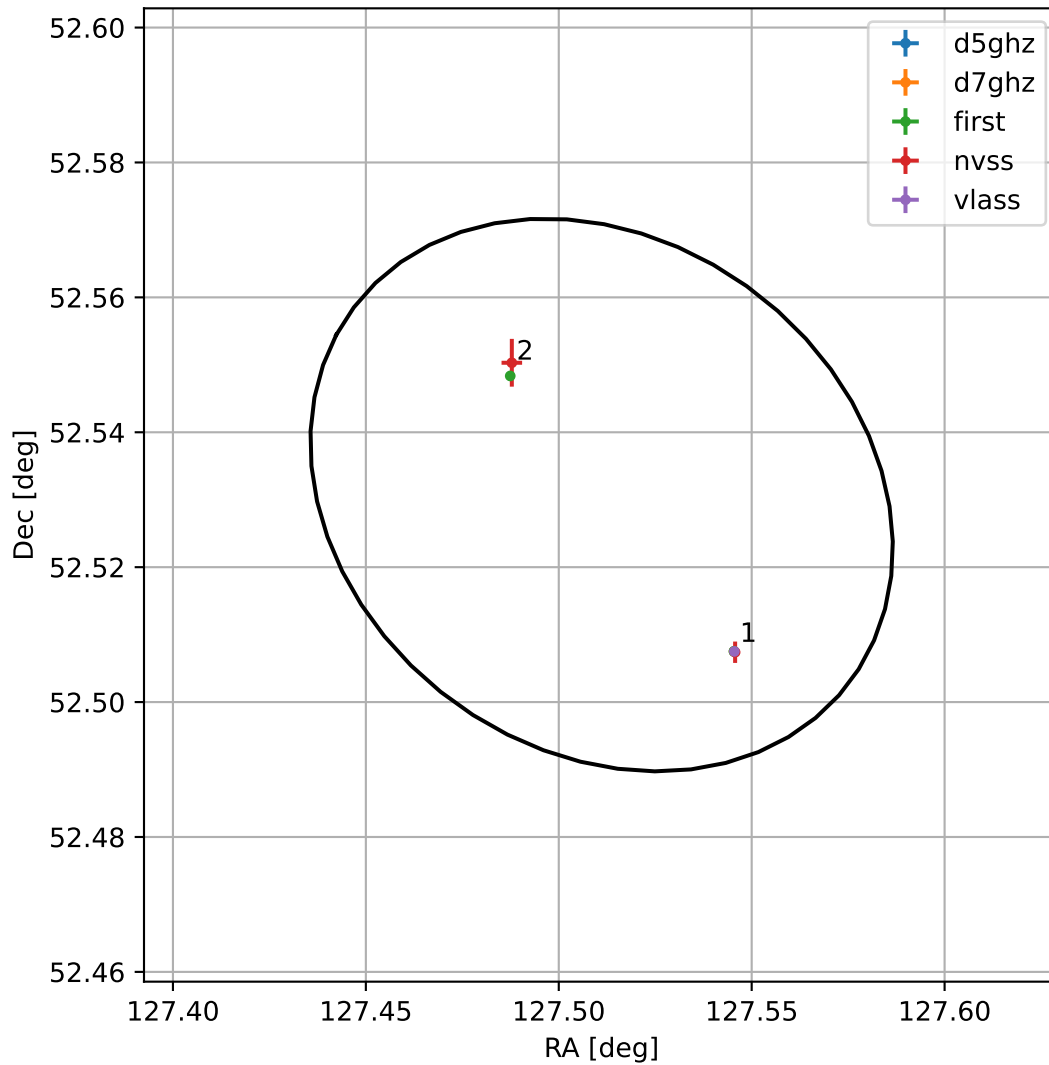
4FGL J0830.0+5231
