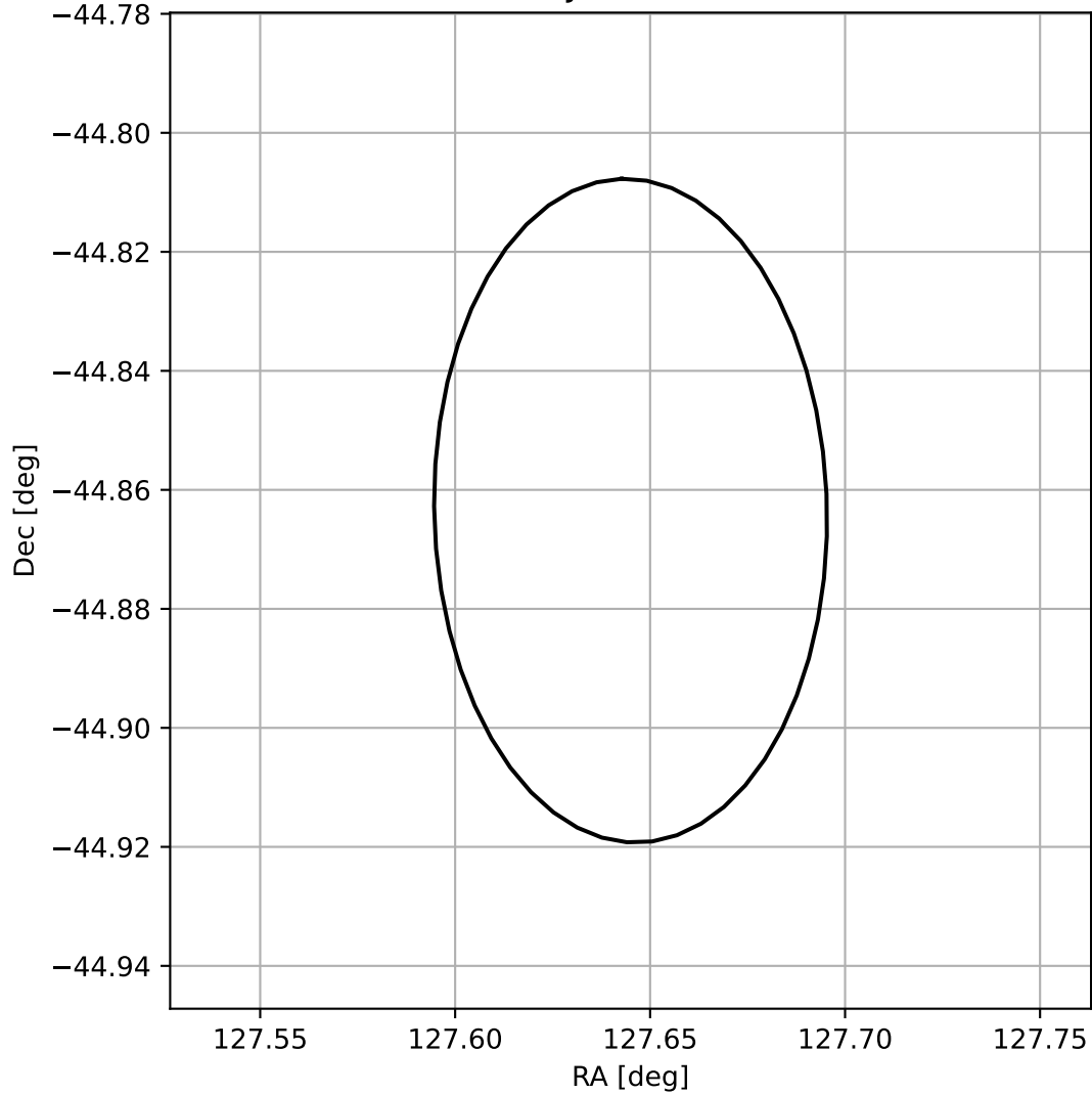
4FGL J0830.5-4451
