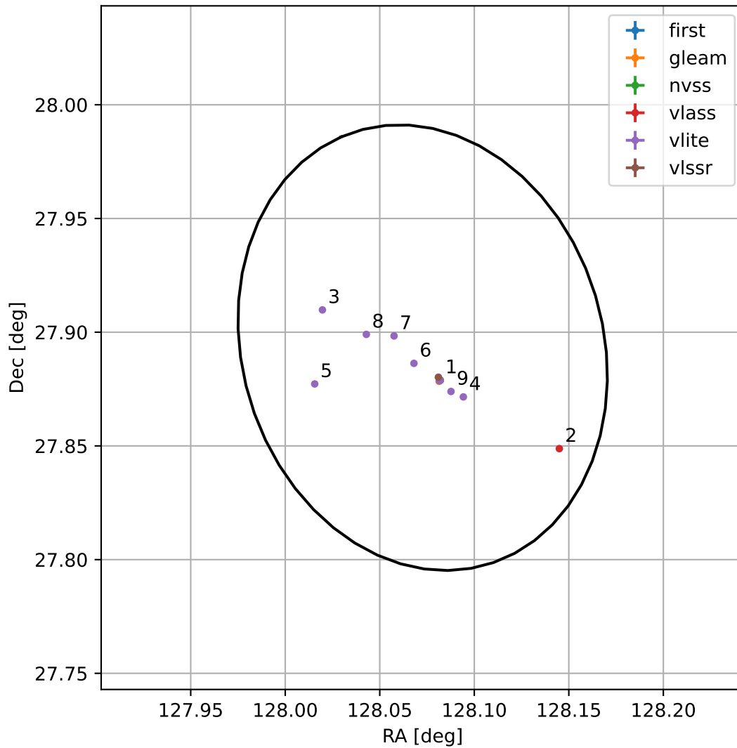
4FGL J0832.2+2753
